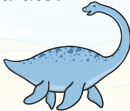
Plesiosaurus
