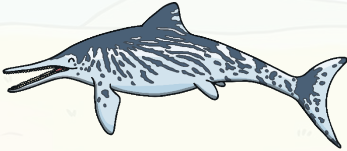
Ichthyosaurus
